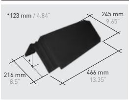
Q145*K | Ridge 45° klinker
