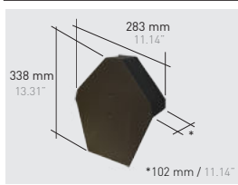
Q147*K | End cap 45° ridge klinker
